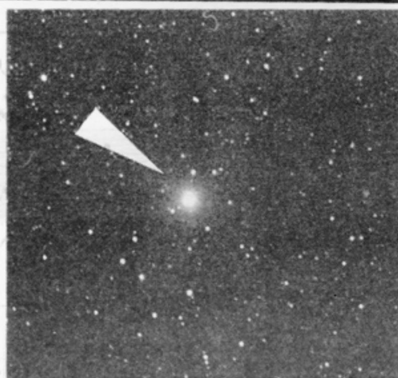
写真 上 1910年5月12日のハレー彗星（ハール天文台） 左下 '85年10月16日 右下 '85年11月8日
